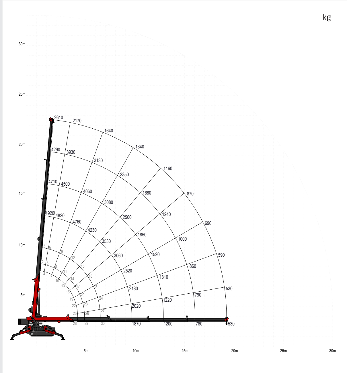
Hauptausleger
